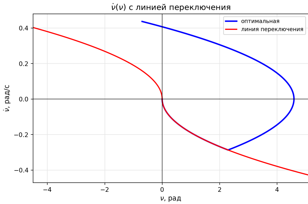
Рис. 5 – Фазовая траектория спутника при моделировании оптимального управления
