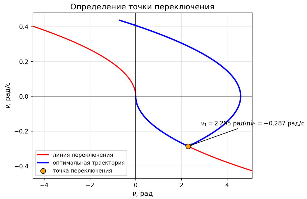
Рис. 4 – Определение точки переключения на фазовой диаграмме
