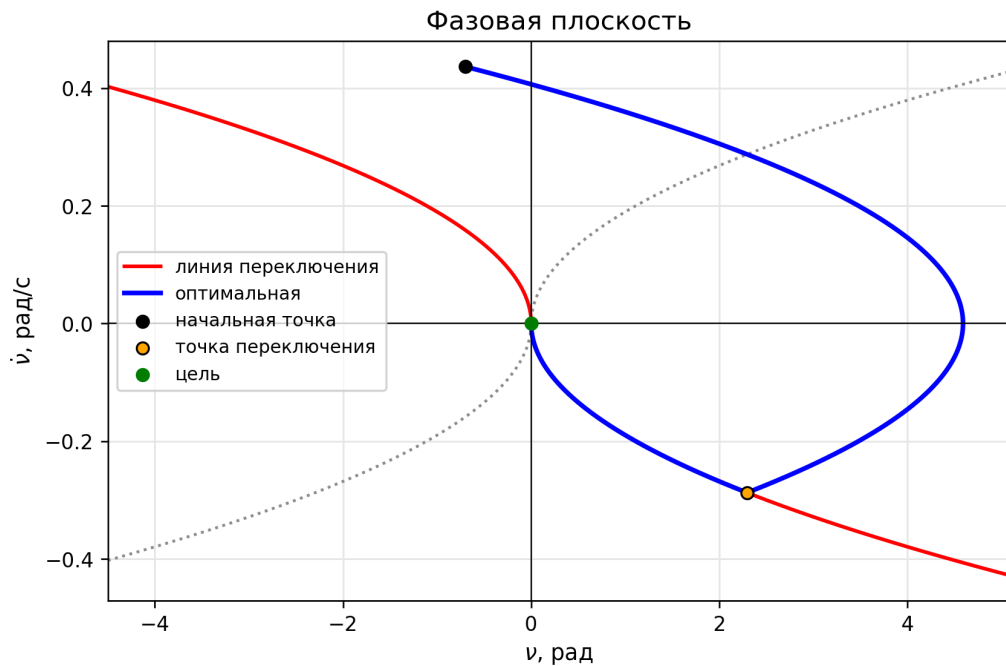
Рис. 3 – Фазовая диаграмма углового движения спутника при оптимальном управлении
