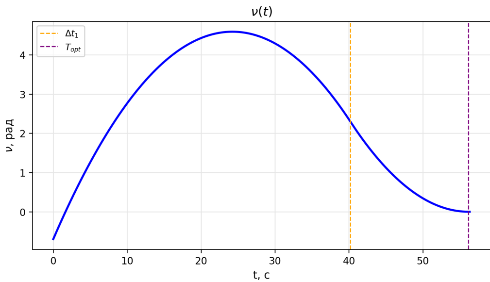
Рис. 6 – График изменения угла \nu(t) при оптимальном управлении
