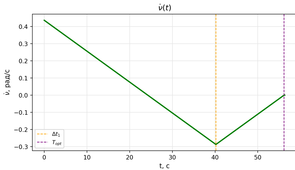
Рис. 7 – График изменения угловой скорости \dot{\nu}(t) при оптимальном управлении
