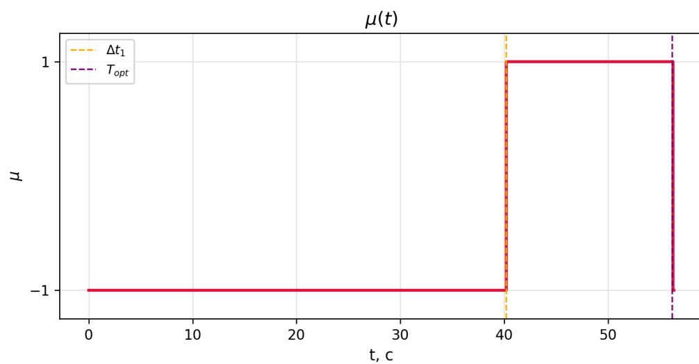
Рис. 8 – График оптимального управляющего воздействия \mu(t)
