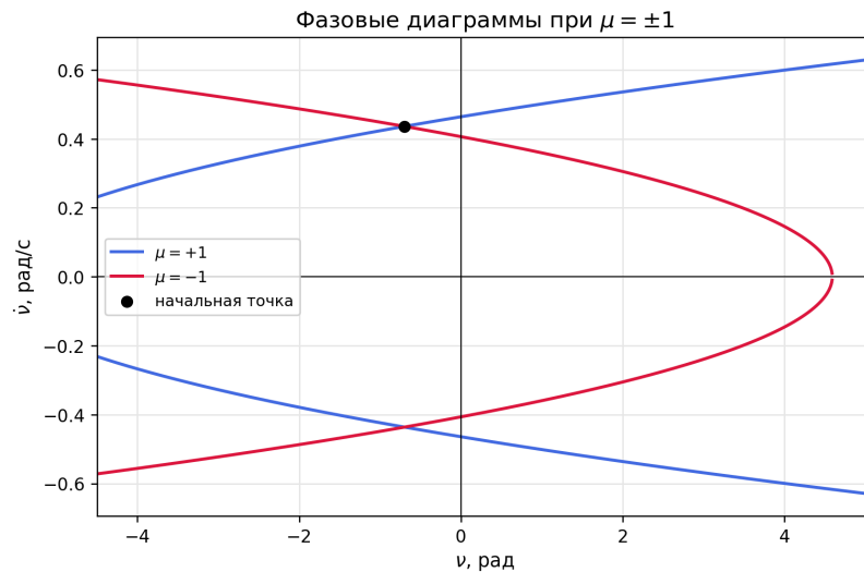
Рис. 2 – Фазовые диаграммы углового движения спутника при \mu = \pm 1
